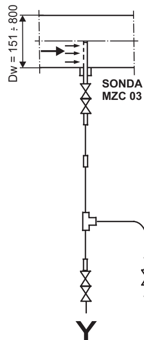
Wykonanie - 02 Czynnik: Para o ciśnieniu do 16 MPa
