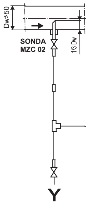
Wykonanie - 01 Czynnik: Woda o ciśnieniu do 22 MPa
