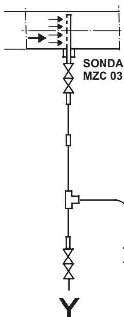
Wykonanie - 02 Czynnik: Para o ciśnieniu do 16 MPa
