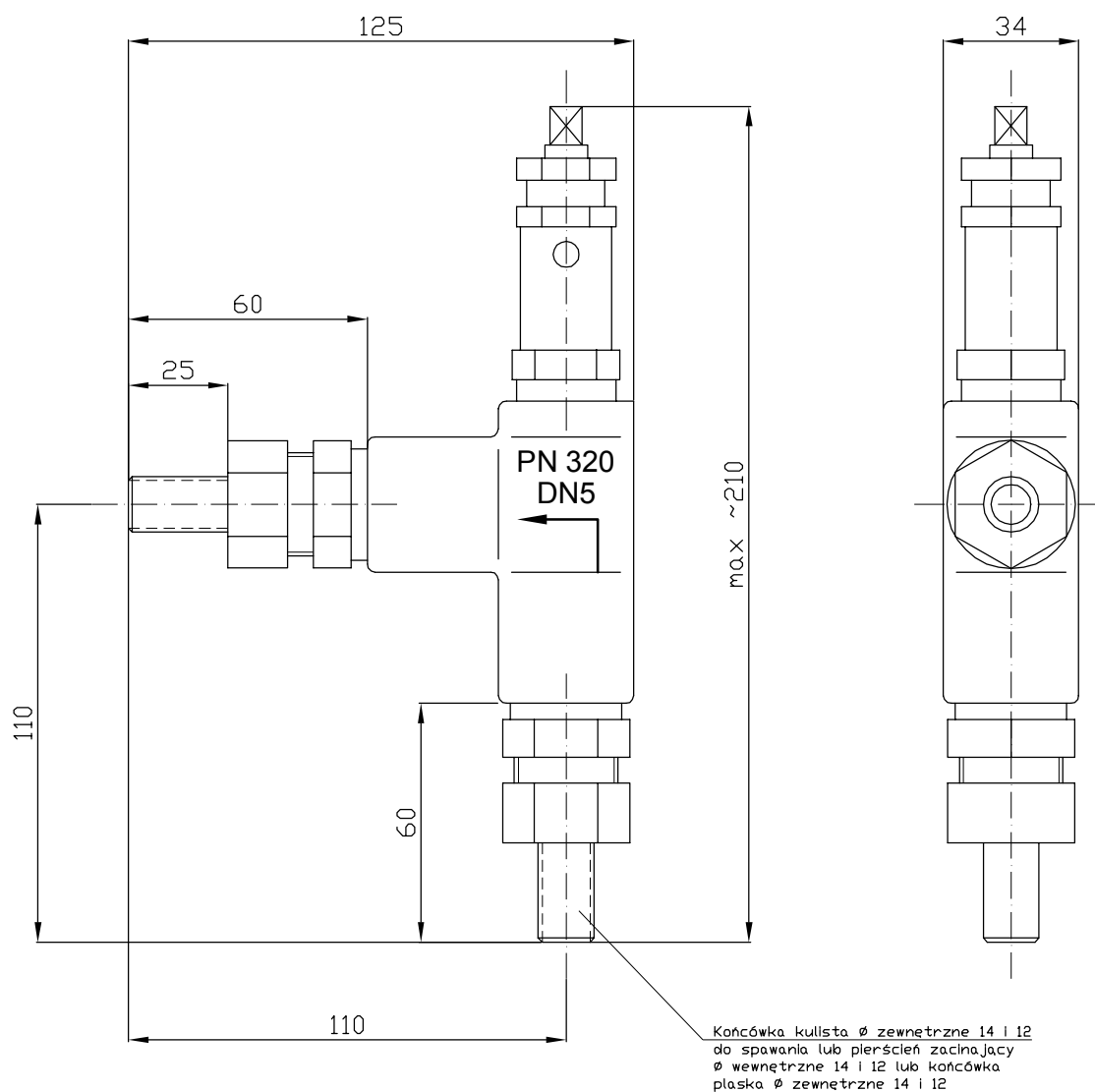
Rys. 1. Zawór jednodrogowy kątowy ZD-MEZ-13-XX/0-0-X
