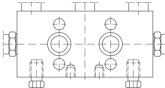
Widok od strony przetwornika
