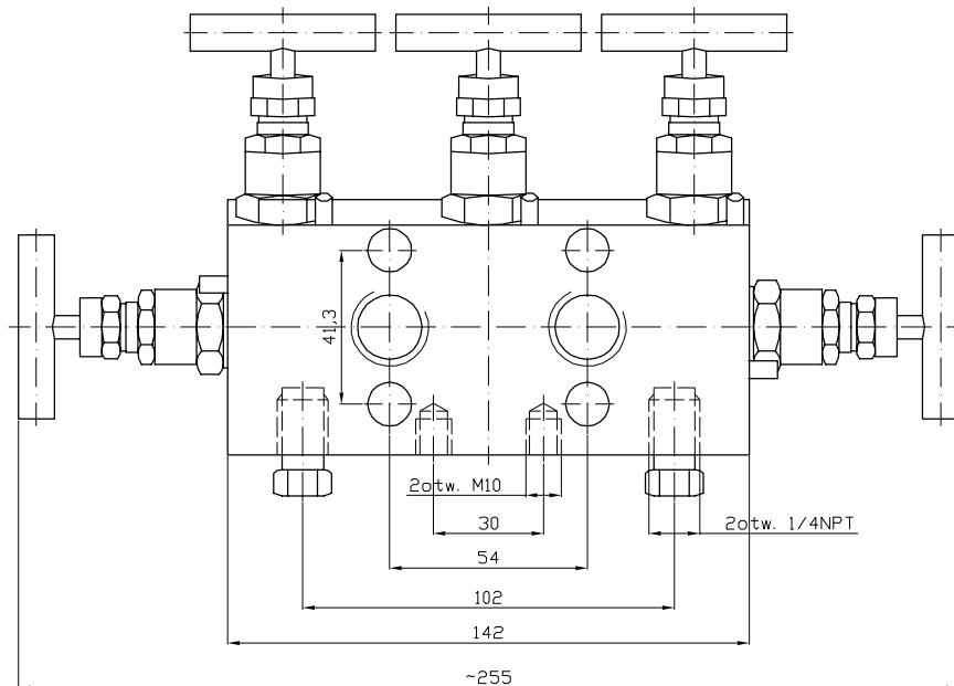
Widok od strony przetwornika
